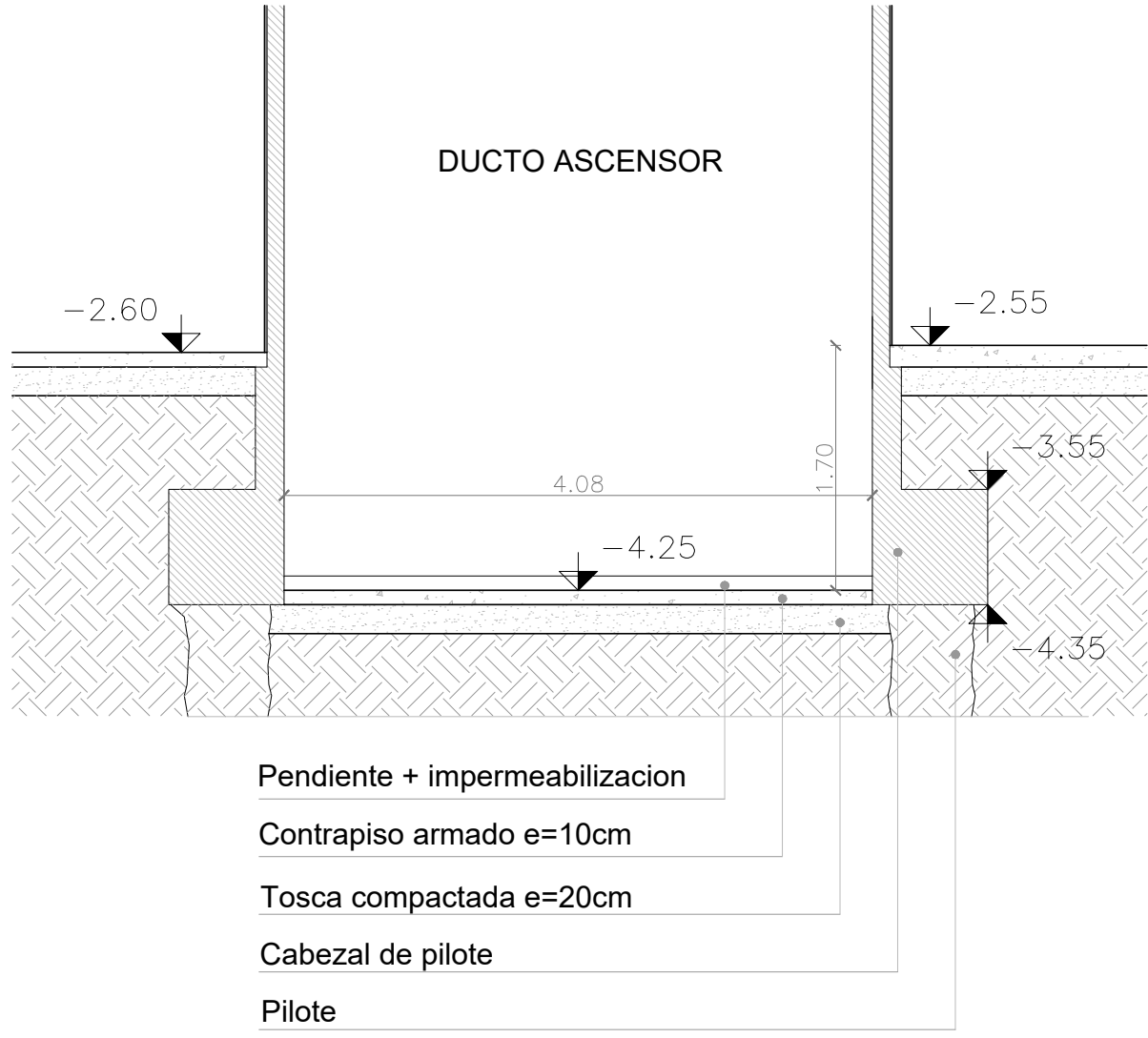
DUCTO ASCENSOR ESC 1/50
